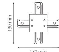
соединитель однофазный встраиваемый X-образный
