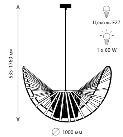
Подвесной светильник
