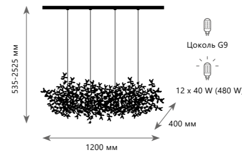
Подвесной светильник
