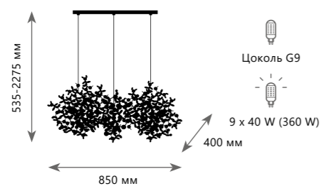
Подвесной светильник
