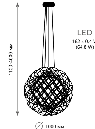
Подвесной светильник
