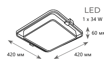
Потолочный светильник
