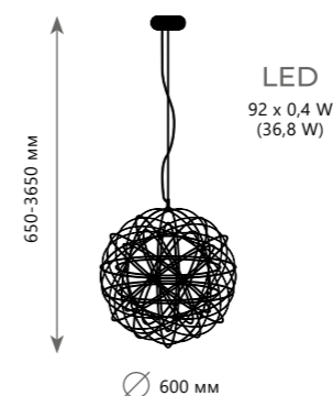
Подвесной светильник
