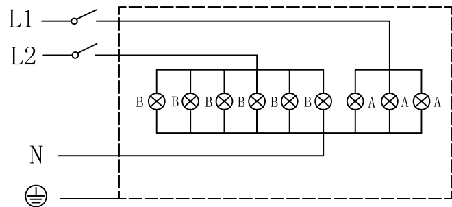
CIRCUIT SCHEMATIC принципиальная (электрическая) схема
