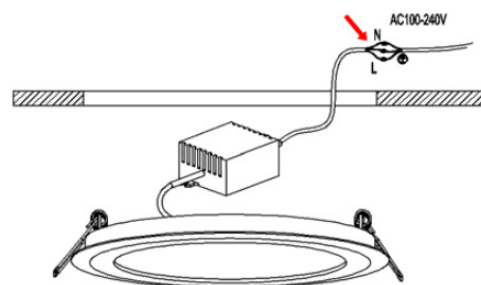
2) подключение led светильника
