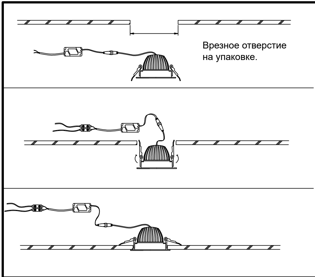
Схема подключения светодиодных светильников (драйвер входит в комплект)
